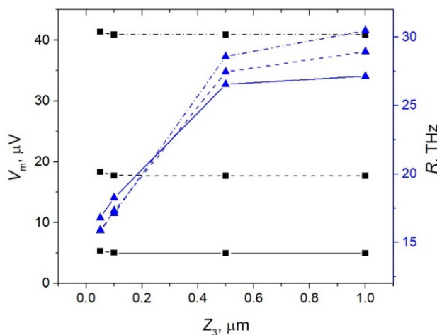
Նկար 4. \text{FeSb}_2 տվիչի վրա առաջացող առավելագույն էլեկտրական լարման ( V_m , քառակուսիներ) և հաշվարկի արագության ( R , եռանկյուններ) կախվածությունը տվիչի հաստությունից ( Z_3 ): Կլանիչի հաստությունն է 0.2 մկմ (անընդհատ գիծ), 0.1 մկմ (կետագիծ) և 0.05 մկմ (կետ-կետագիծ) [16]:
