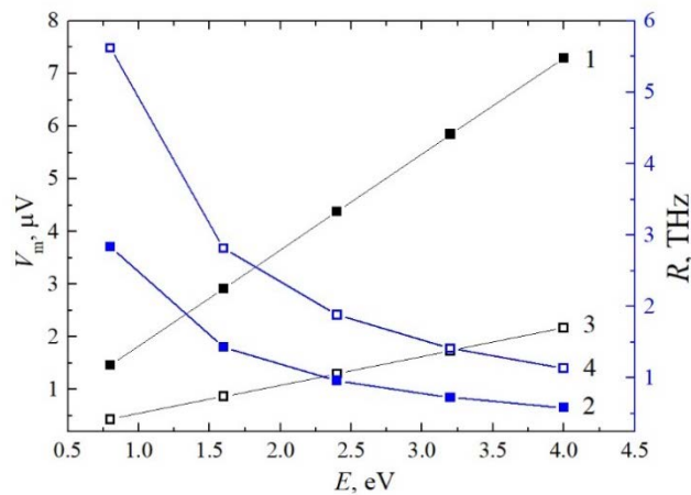
Նկար 3. V_m(1, 3) և R(2, 4) բնութագրերի կախվածությունը ֆոտոնի էներգիայից. կլանիչի հաստությունը Z_2=0.1 մկմ (1, 2) և Z_2=0.2 մկմ (3, 4) [14]:
