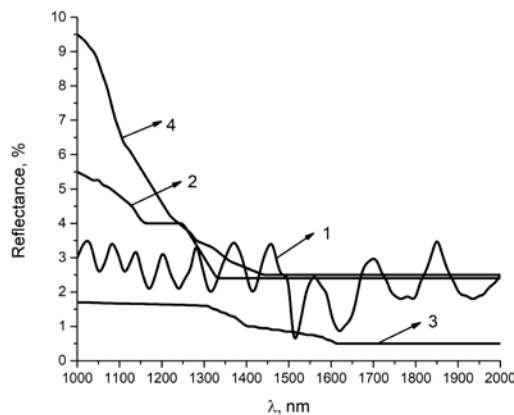
Նկար 8. \text{SiO}_2 թաղանթների անդրադարձման սպեկտրերը. ( \text{Al}_2\text{O}_3 տակդիր՝ 1 – \text{SiO}_1\text{a}_2 , 2 – \text{SiO}_2\text{a}_3 , 3 – \text{SiO}_3\text{a}_3 և \text{AlN} տակդիր՝ 4 – \text{SiO}_2\text{b}_3 ) [21]:
