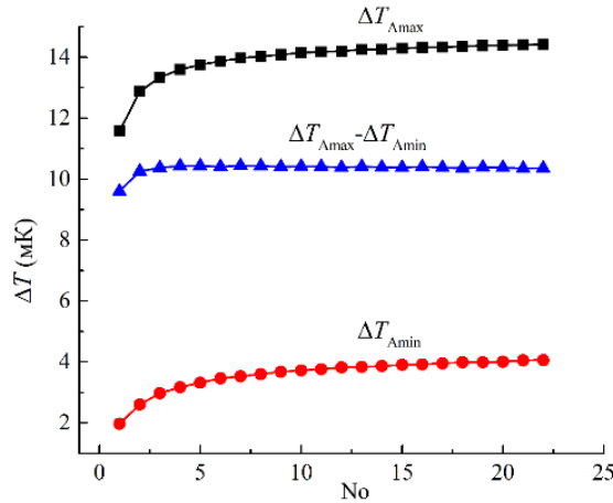
Նկար 7. \Delta T_{\text{Amax}} , \Delta T_{\text{Amin}} և \Delta T_{\text{Amax}} - \Delta T_{\text{Amin}} պարամետրերի կախվածությունը կլանված ֆոտոնի համարից 0.005 պվ ժամանակային հապաղման դեպքում [19]:
