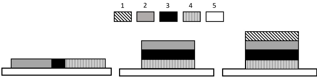
Նկար 1. ՋՄՖԴ զգայուն տարրի կառուցվածքը. միաշերտ, եռաշերտ և քառաշերտ: 2զայուն տարրի շերտեր. 1 - հակաանդրադարձնող, 2 - կլանիչ, 3 - տվիչ, 4 - ջերմատար, 5 - տակդիր:
