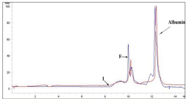
Գծապատկեր 1. Առնետի շիճուկային ալբումինի (RSA-ի) (0.25 մգ/մլ ջրային լուծույթ) էլեկտրոֆորեզրաման՝ բաժանված 48.5սմ/50մկմ մերկ ծուլված կվարցային մազանոթով: Մազանոթային էլեկտրոֆորեզի ընթացքի պարամետրեր. 30 մմոլ/լ pH=9.5 Բորատային բուֆեր, 15կվ լարում, 20°C ջերմաստիճան, 450 մԲար/վրկ ներարկում, 200նմ ալիքի երկարություն:
