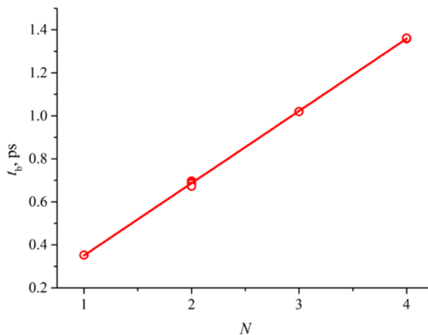
Նկար 6. t_b -ի կախվածությունը միաժամանակ կլանված ֆոտոնների թվից [18]:
