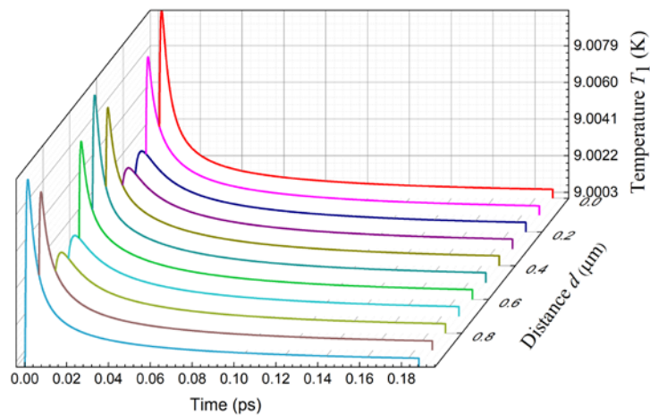
Նկար 5. Կլանիչ-տվիչ սահմանի ջերմաստիճանի տարածա-ժամանակային կախվածությունը [17]:
