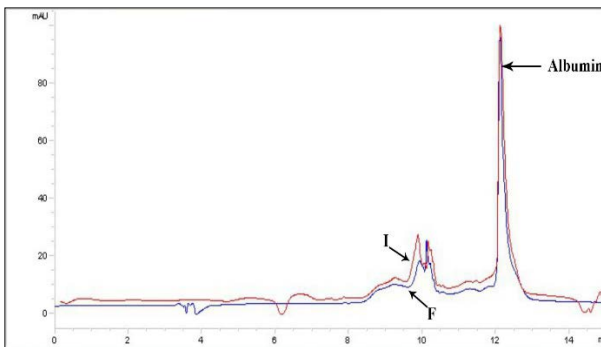
Գծապատկեր 1. Առնետի շիճուկային ալբումինի (RSA-ի) (0.25 մգ/մլ ջրային լուծույթ) էլեկտրոֆորեզրաման՝ բաժանված 48.5սմ/50մկմ մերկ ծուլված կվարցային մազանոթով: Մազանոթային էլեկտրոֆորեզի ընթացքի պարամետրեր. 30 մմոլ/լ pH=9.5 Բորատային բուֆեր, 15կվ լարում, 20°C ջերմաստիճան, 450 մԲար/վրկ ներարկում, 200նմ ալիքի երկարություն:
