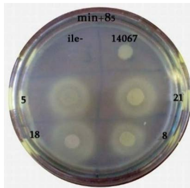
Նկար 2. Տրիպտոֆանի սինթեզի գնահատումը թեստ-կուլտուրայի կիրառմամբ: (տր Թեստ-կուլտուրա պարունակող Գլովերի միջավայր)
