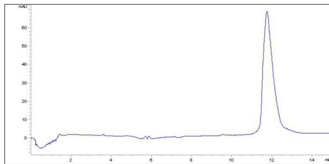
Գծապատկեր 1. Առնետի շիճուկային ալբումինի (RSA-ի) (0.25 մգ/մլ ջրային լուծույթ) էլեկտրոֆորեզրաման՝ բաժանված 48.5սմ/50մկմ մերկ ծուլված կվարցային մազանոթով: Մազանոթային էլեկտրոֆորեզի ընթացքի պարամետրեր. 30 մմոլ/լ pH=9.5 Բորատային բուֆեր, 15կվ լարում, 20°C ջերմաստիճան, 450 մԲար/վրկ ներարկում, 200նմ ալիքի երկարություն:
