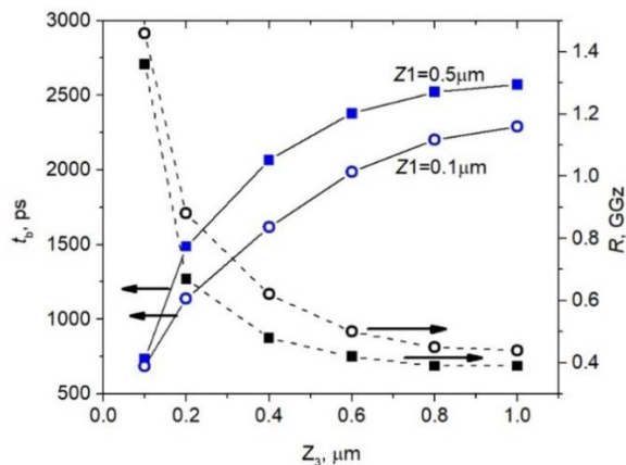
Նկար 2. ԶՄՖԴ-ի քառաշերտ զգայուն տարրի t_b և R բնութագրերը [13]:
