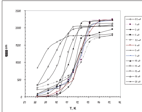
Նկ.1. Չափման հոսանքի մեծության ազդեցությունը տեսակարար դիմադրության ջերմաստիճանային կախվածության վրա:
