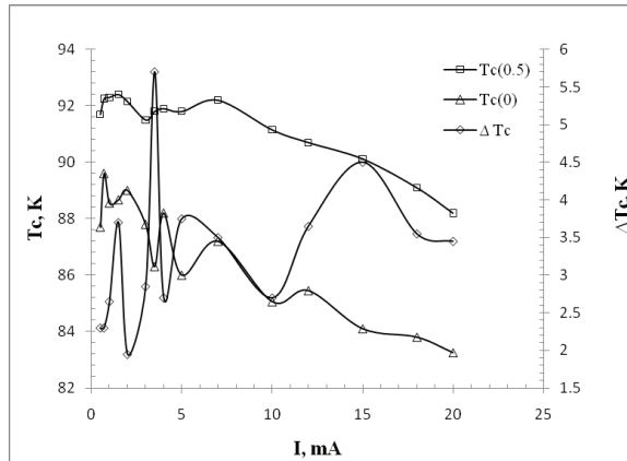
Նկ. 3. Գերհաղորչային անցման լայնության \Delta T_c , ինչպես նաև T_c(0) և T_c(0.5) կրիտիկական ջերմաստիճանների կախվածությունը չափման հոսանքի մեծությունից:
