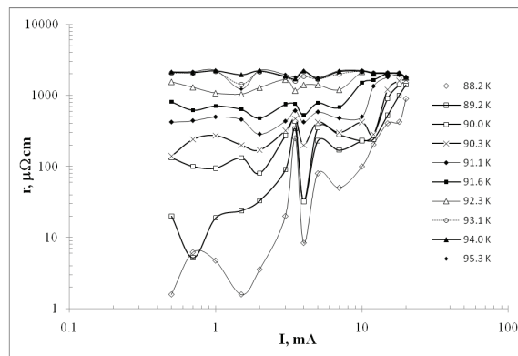
Նկ. 2. Տեսակարար դիմադրության կախվածությունը չափման հոսանքից տարբեր ջերմաստիճանների համար:
